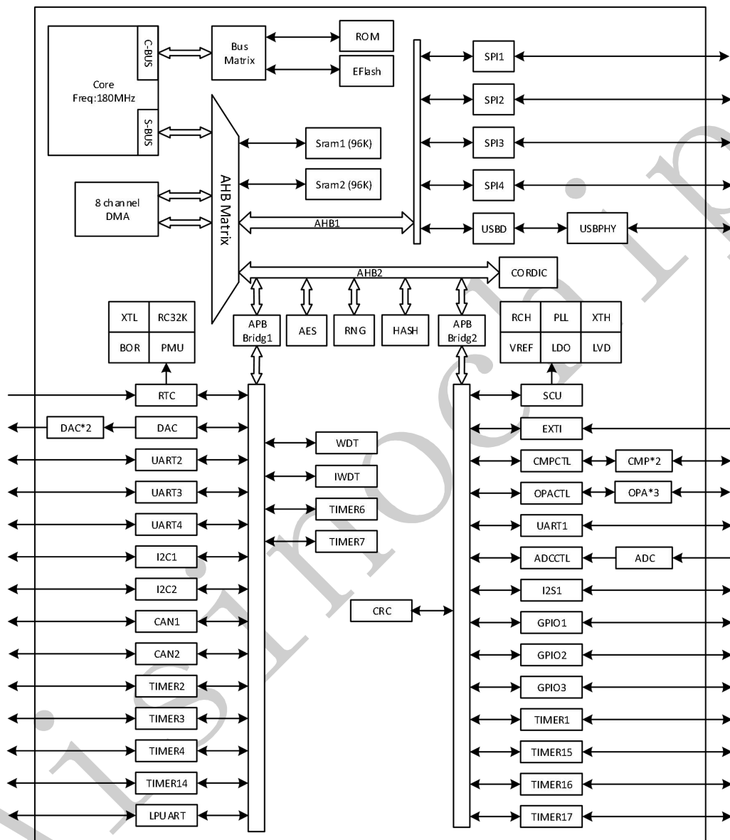
图 3-1 ACM32F403 功能框图
