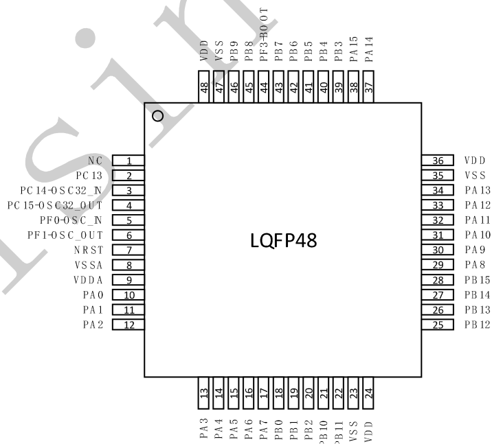
图 4-3 LQFP48 封装管脚分布图
