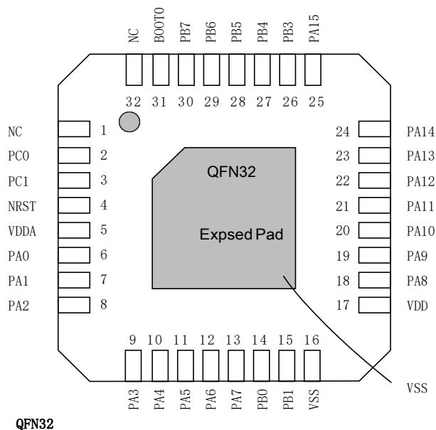
图 2-2 QFN32 封装管脚排布图
