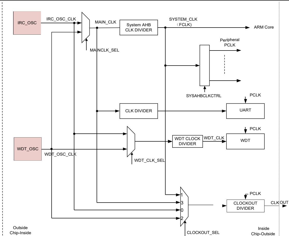
图 4-3 时钟树
