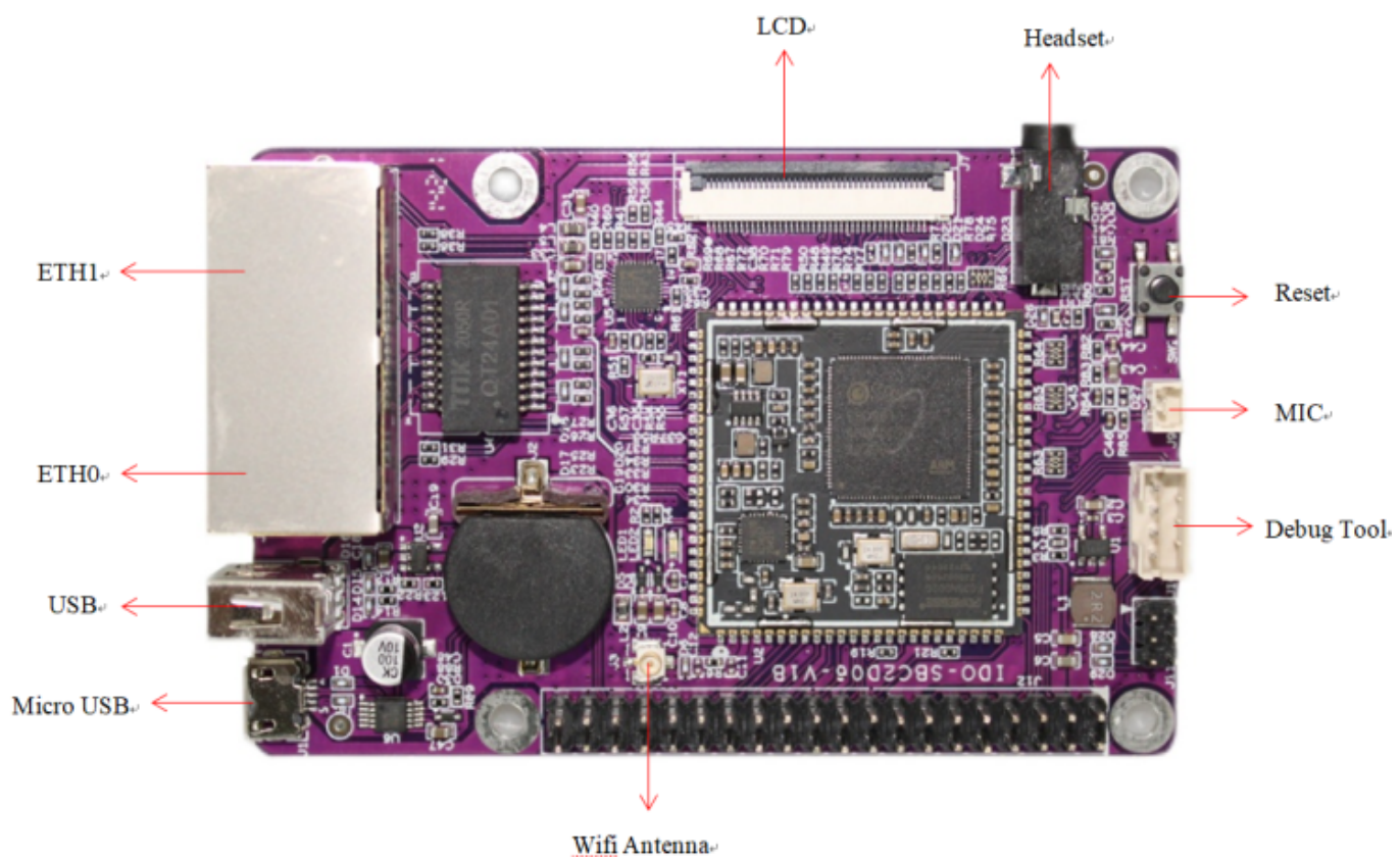
开发板正面
