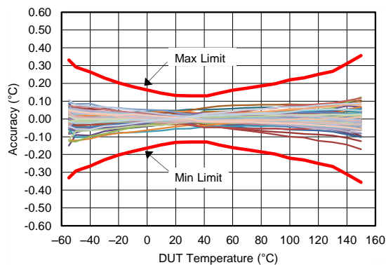
LMT70 精度与温度间的关系
