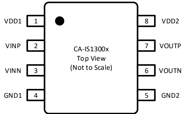
图 6-1 CA-IS1300x 引脚配置
