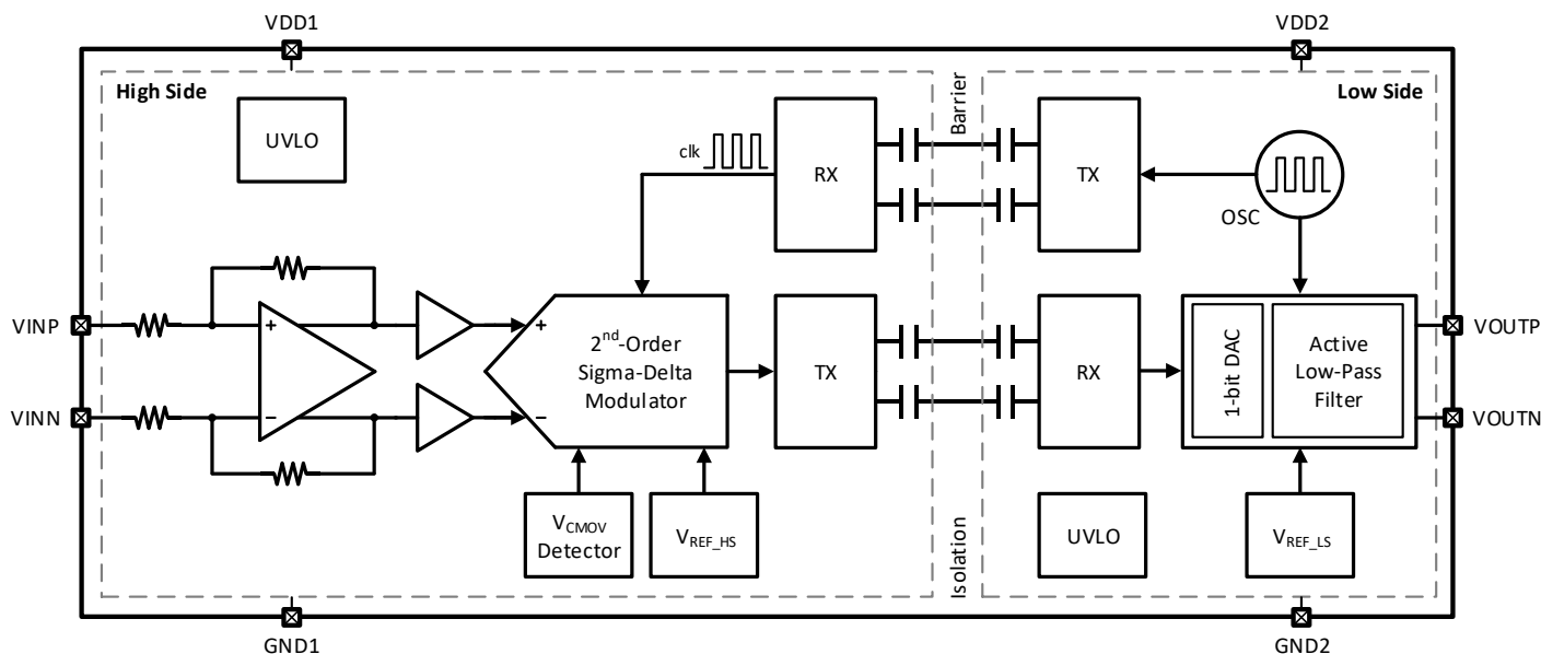
图 9-1 CA-IS1300x 功能框图
