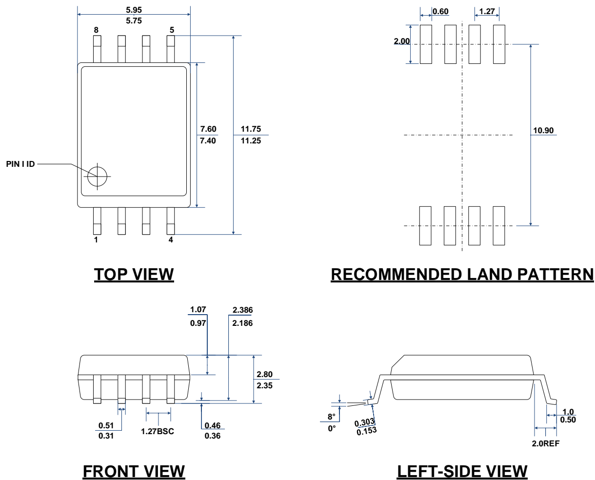
图 11-1 SOIC8 宽体封装外形尺寸图
