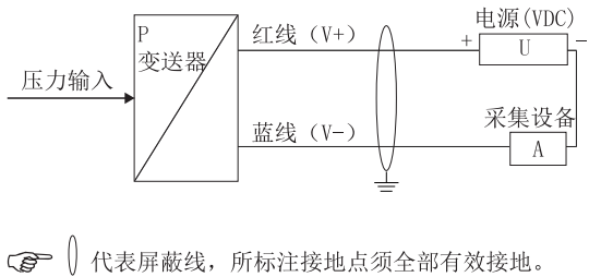
电流输出接线图（两线制）
