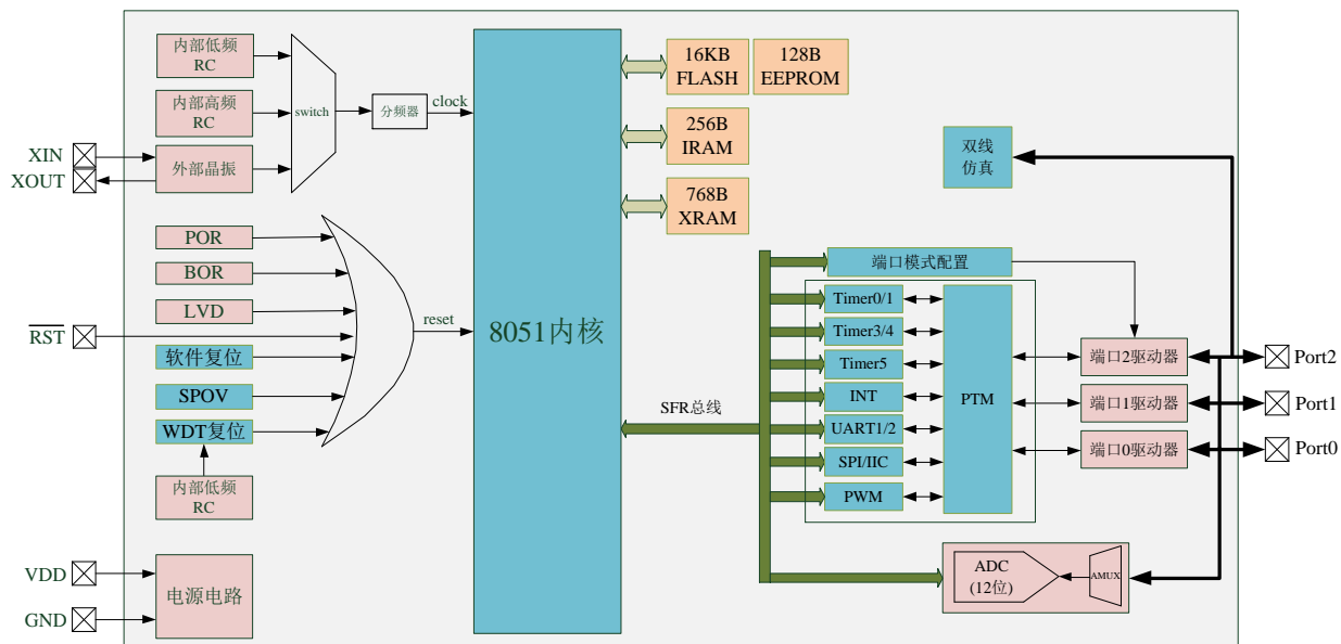
Figure 1-1 系统框图
