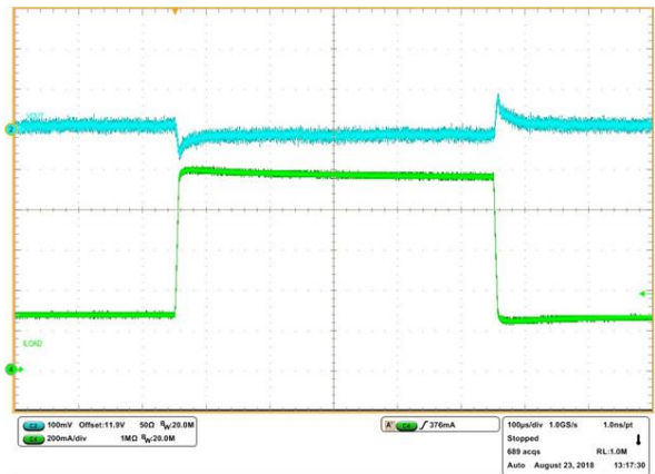
图 16. Load Step Response
