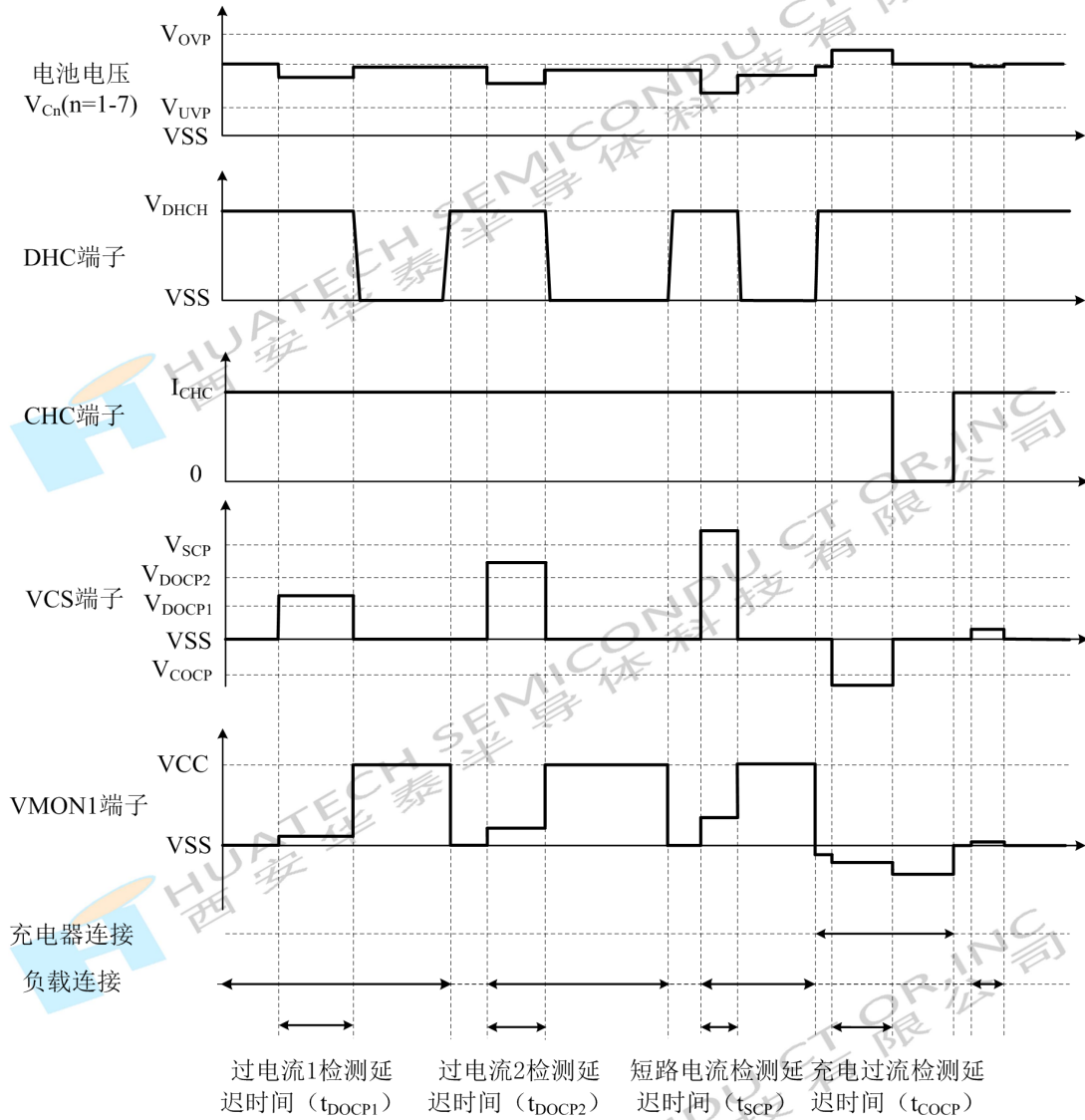
图9 放电过流检测、充电过流检测
