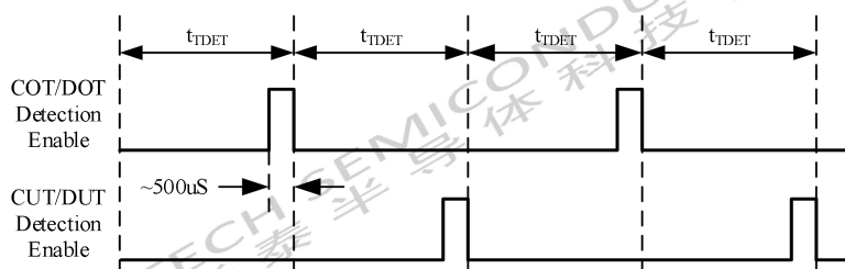
图 7 温度检测时序
