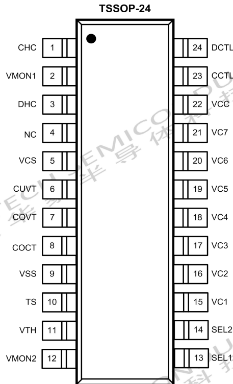
图 5 管脚分布
