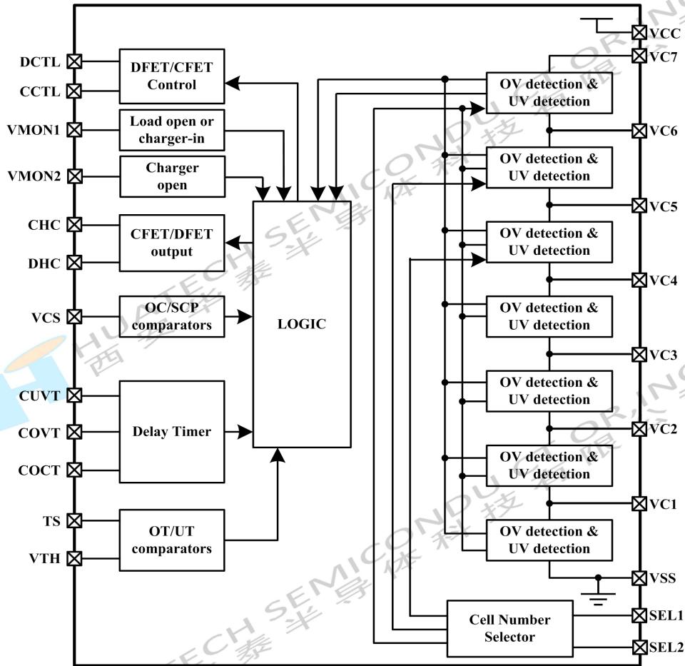
图 6 功能框图
