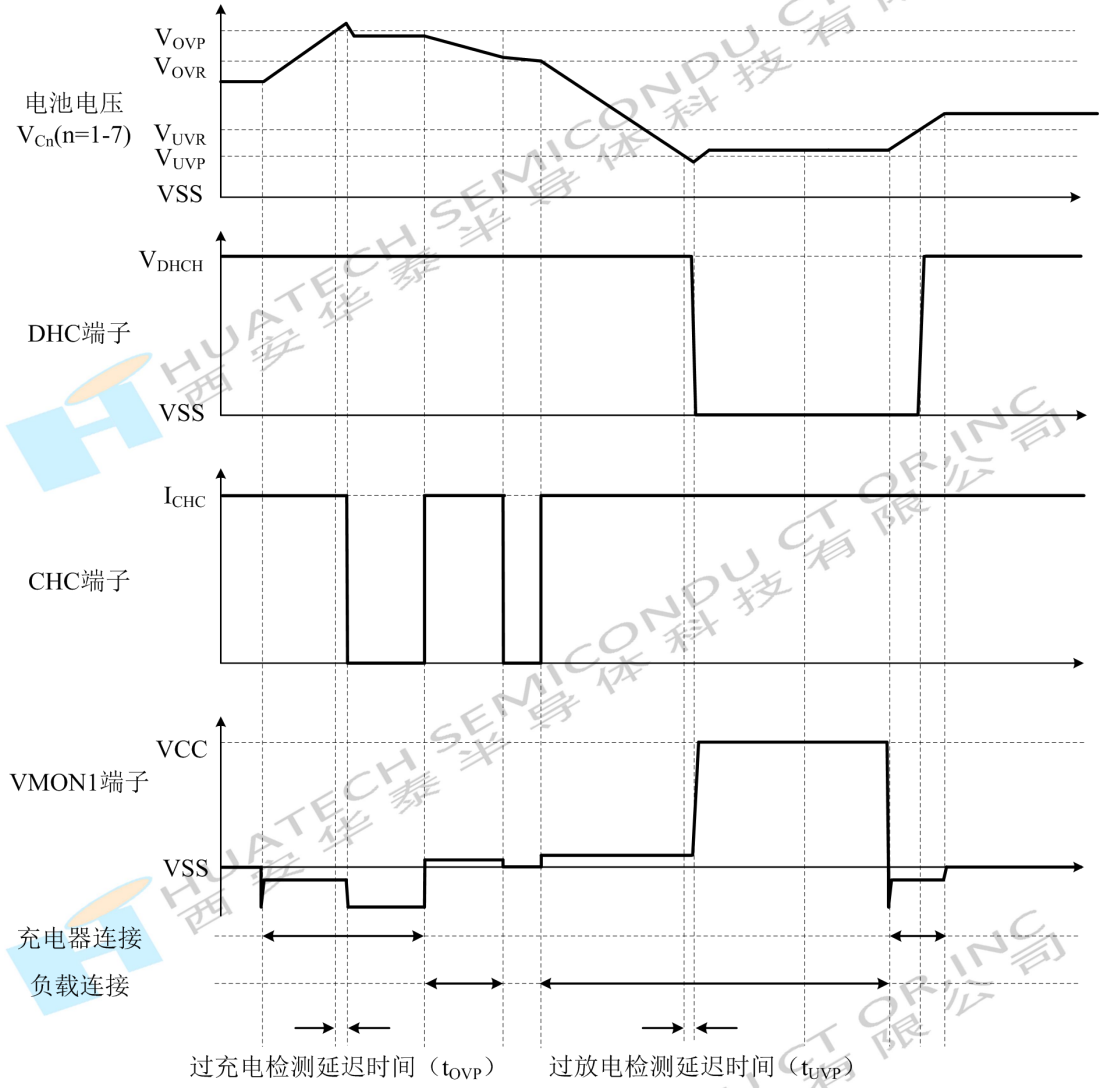
图 8 过充电检测、过放电检测
