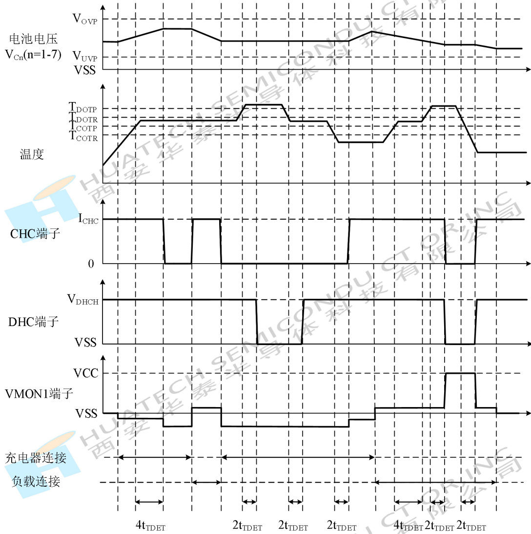
图 11 充放电高温检测
