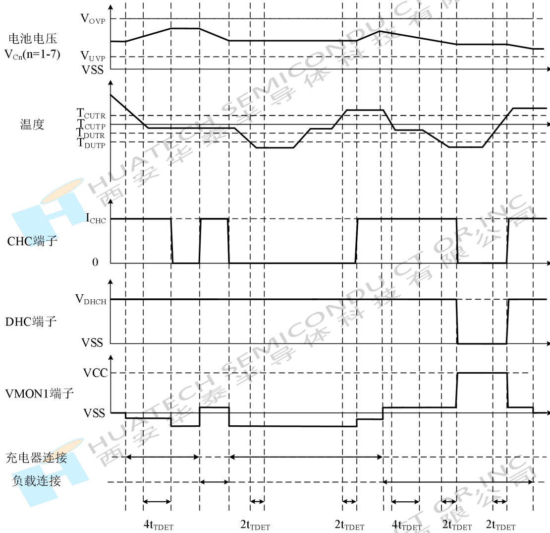
图 12 充放电低温检测
