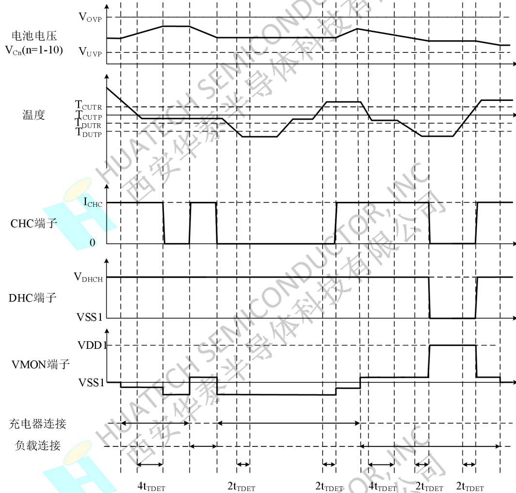
图 10 充放电低温检测
