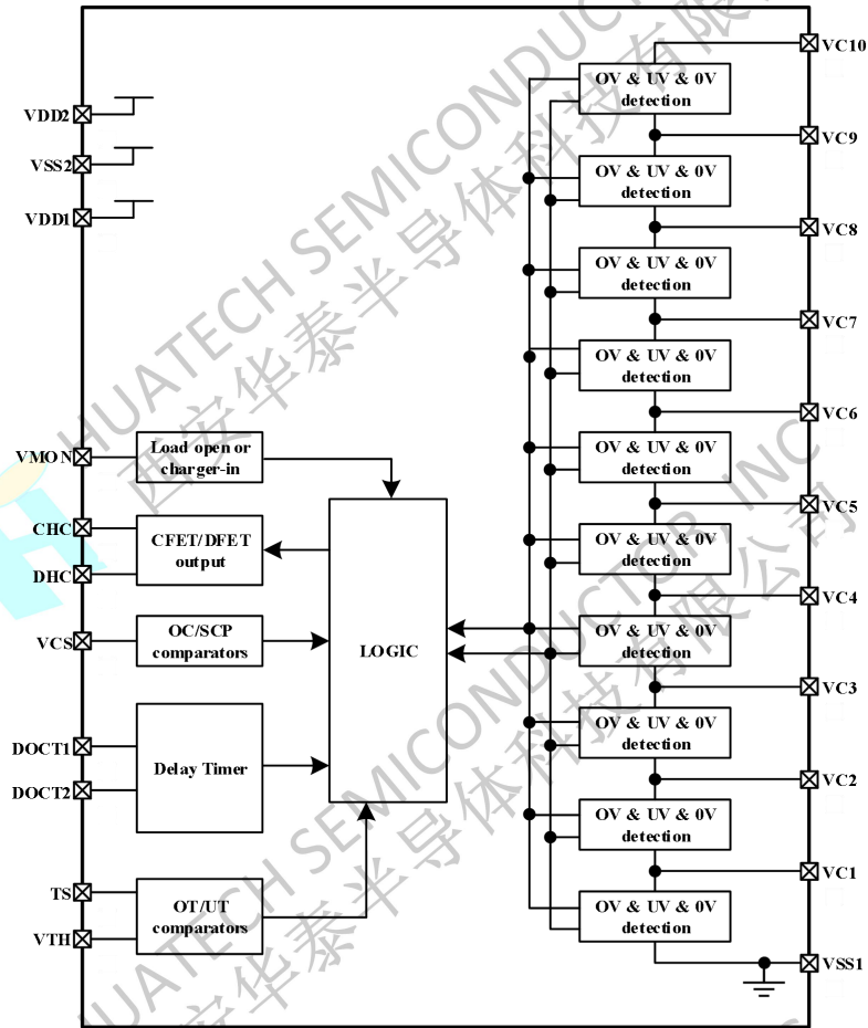
图 4 功能框图
