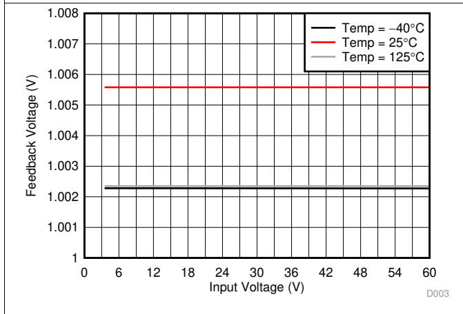
图 3. Feedback Voltage
