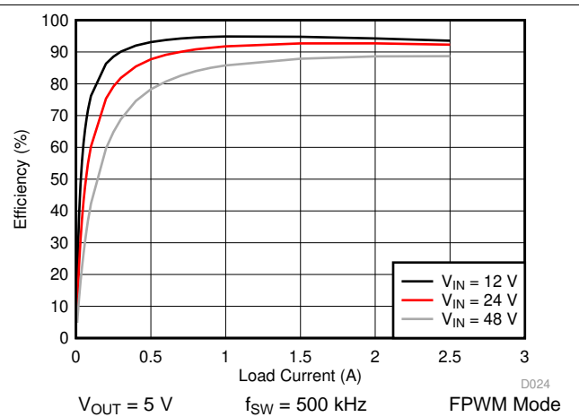
图 36. LM76002 Efficiency
