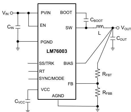
简化原理图
