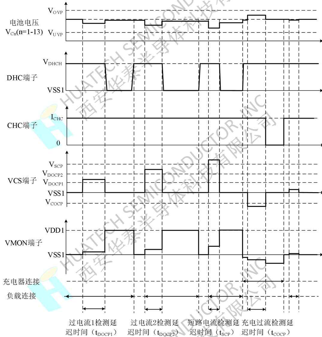
图 8 放电过流检测、充电过流检测
