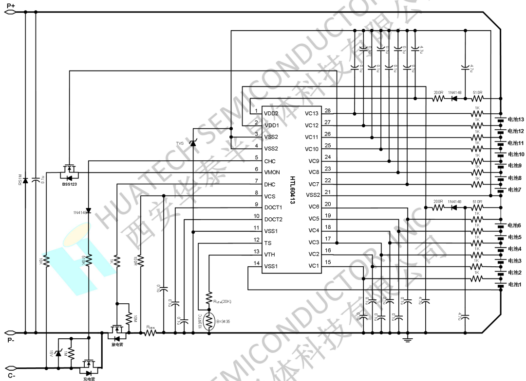
图 2 13 节电池包的 N 型充电管和 N 型放电管的 C-分口典型应用电路图
