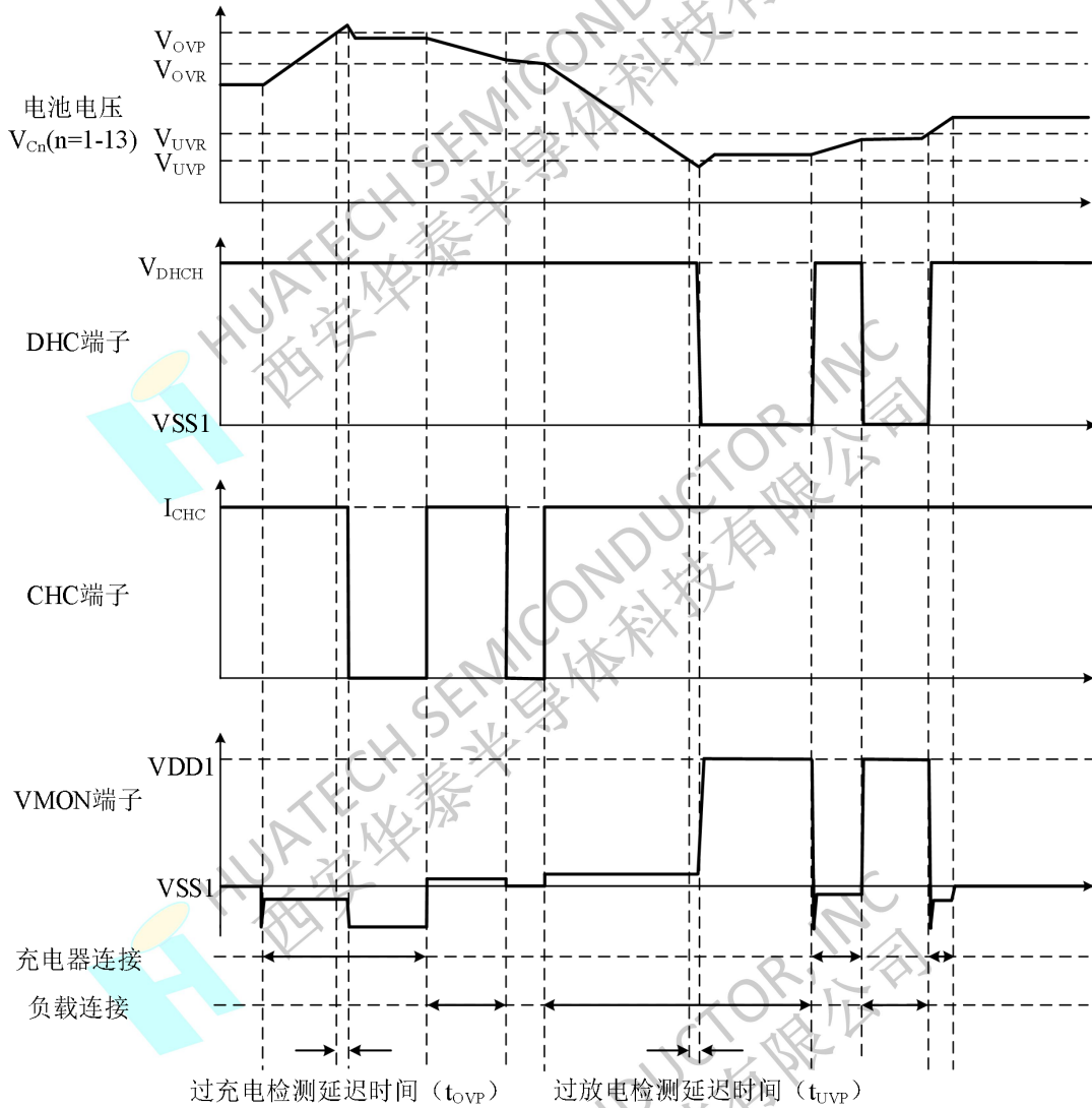
图 7 过充电检测、过放电检测
