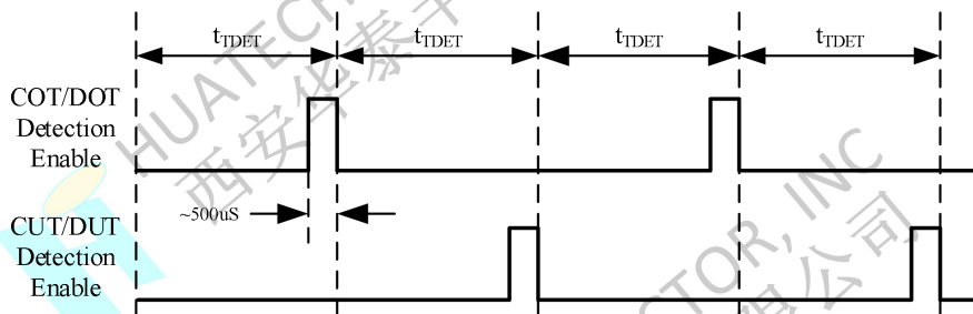
图 5 温度检测时序
