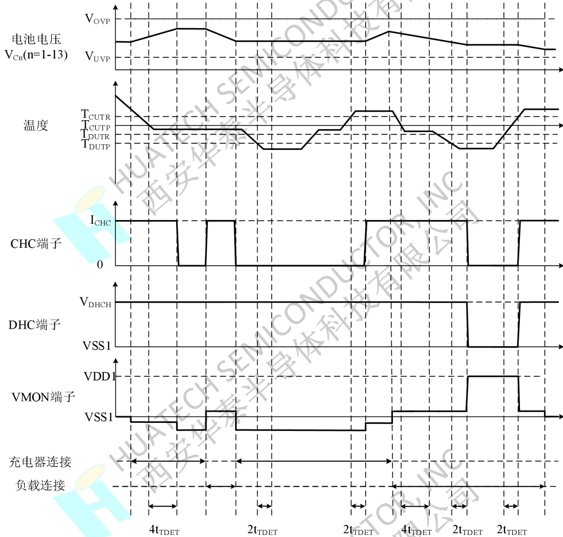
图 10 充放电低温检测
