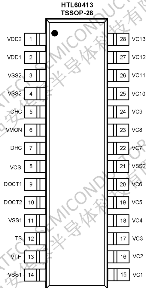
图 3 引脚分布
