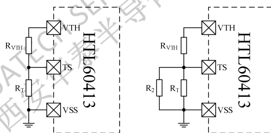
图 6 (a) R_{VTH} + R_T 方式 (b) R_{VTH} + R_T \parallel R_2 方式
