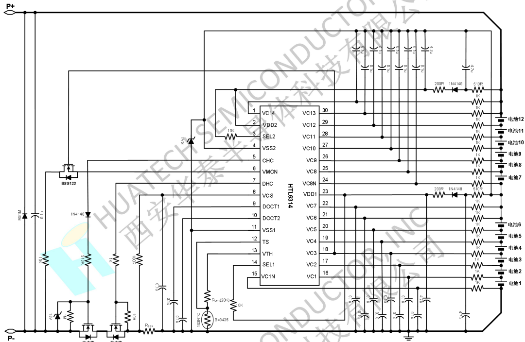
图 4 12 节电池包的 N 型充电管和 N 型放电管的同口典型应用电路图
