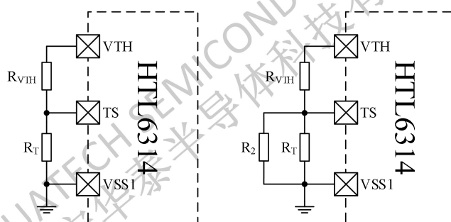
图 13 (a) R_{VTH}+R_T 方式
