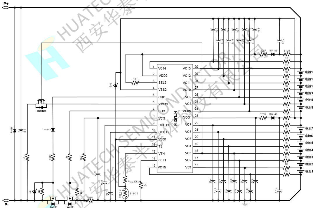
图 3 13 节电池包的 N 型充电管和 N 型放电管的同口典型应用电路图
