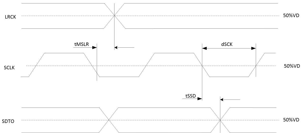
音频接口时序（主机模式）
