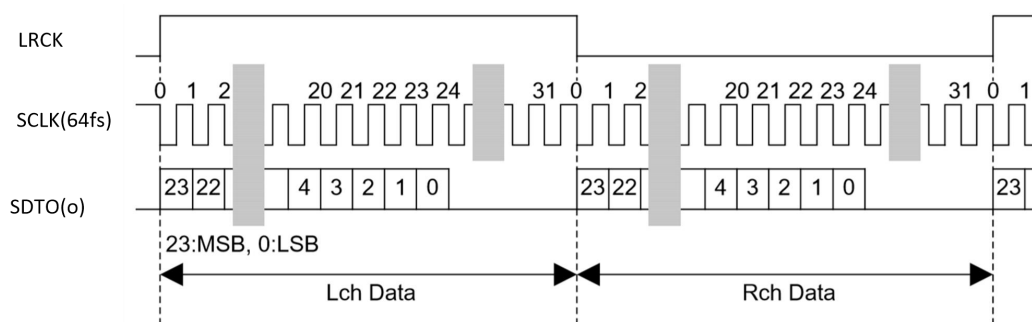
图 1. Mode 0 时序
