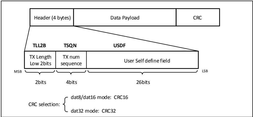
图10-2 数据包格式
