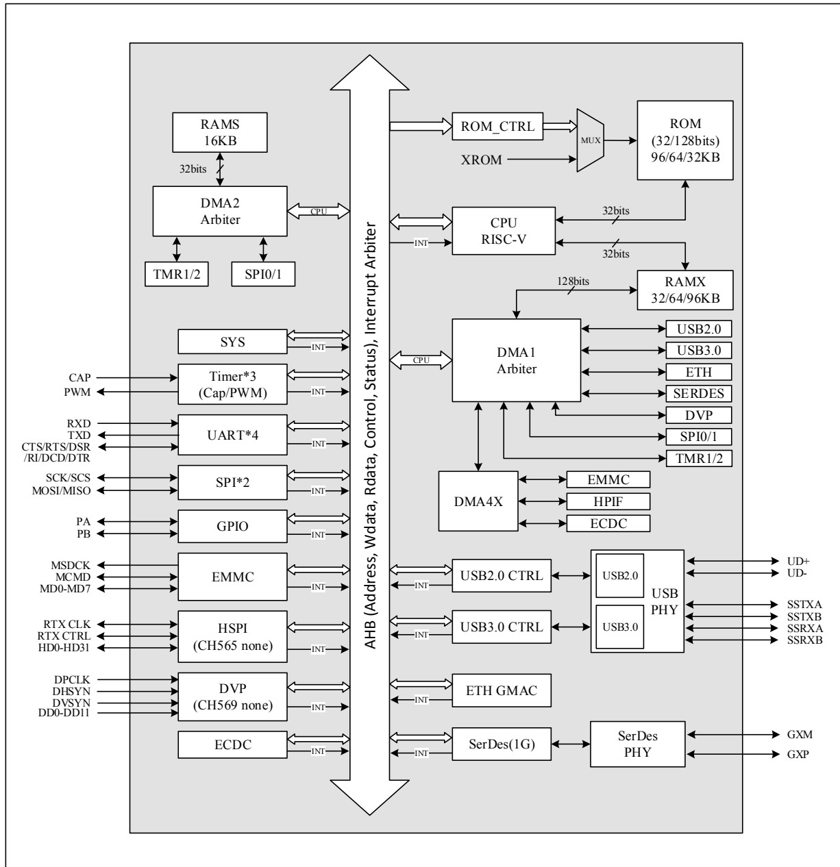
图 2-1 系统框图
