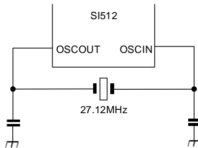
图 15.1 晶振连接
