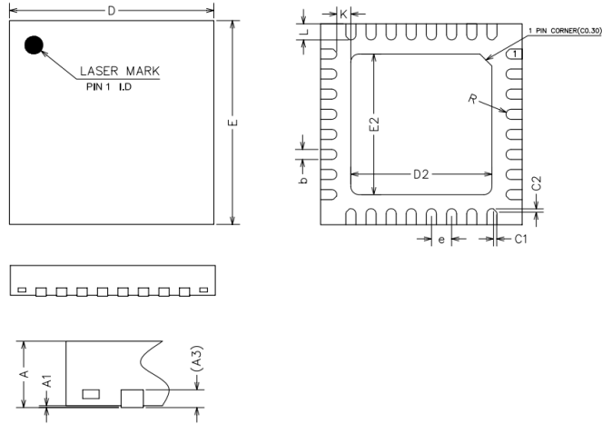
图 20.1 Si512 封装示意图
