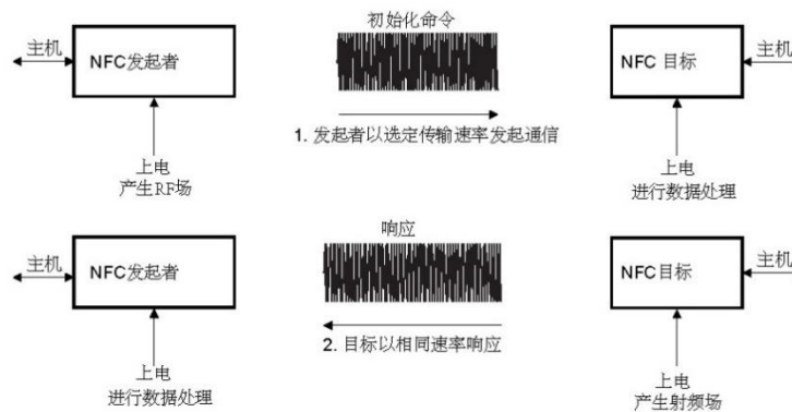
图 6.7 主动通信模式
