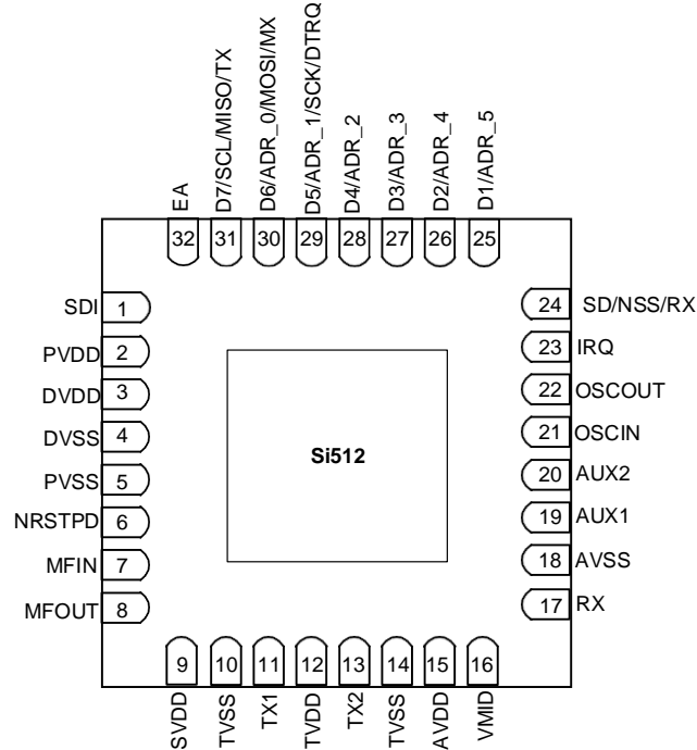
图 5.1 Si512 管脚示意图
