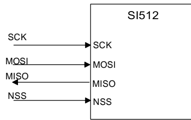
图 8.1 SPI 接口
