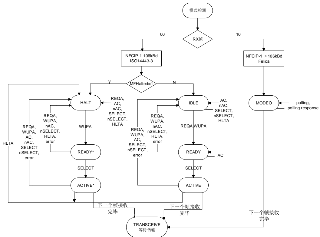
图 17.1 AutoColl 命令
