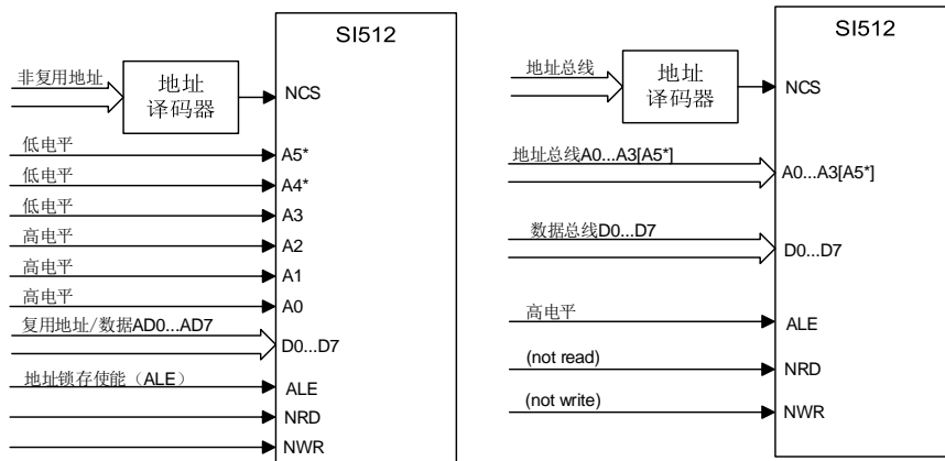
图 9.1 分立读写时与主机控制器连接
