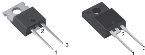
TO-220AC
