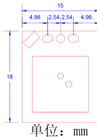
图 4.2 MW5L15-B 模块尺寸图
