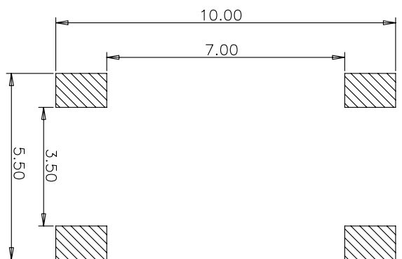
RECOMMENDED P.C.B. LAYOUT 安装尺寸图
