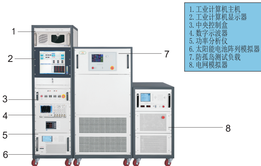
TPVS1000 测试系统控制平台
