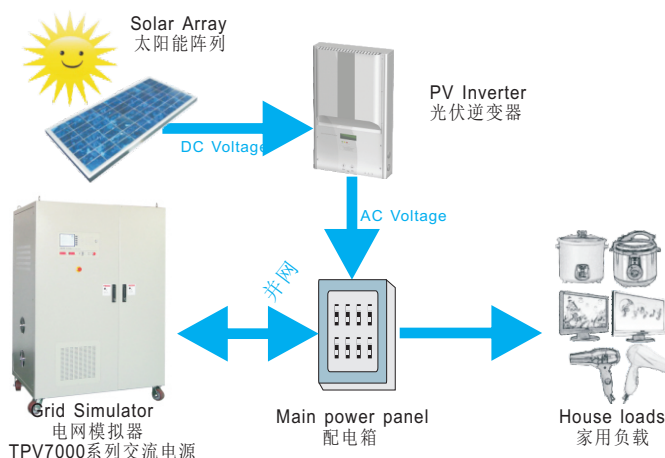
用TPV7000系列交流电源模拟电网示意图
