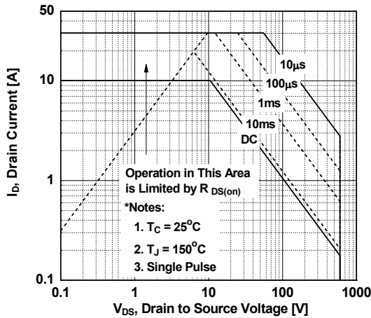
图 9. 最大安全工作区 (FCP380N60E)
