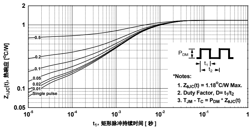
图 14. 瞬态热响应曲线 (FCPF380N60E)
