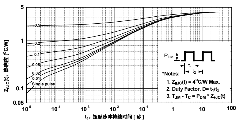
图 14. 瞬态热响应曲线 (FCPF380N60E)
