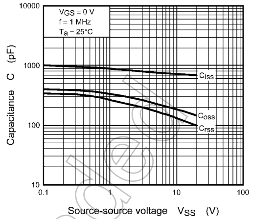
Fig. 10.8 Capacitance - V_{SS} (Note 5)
