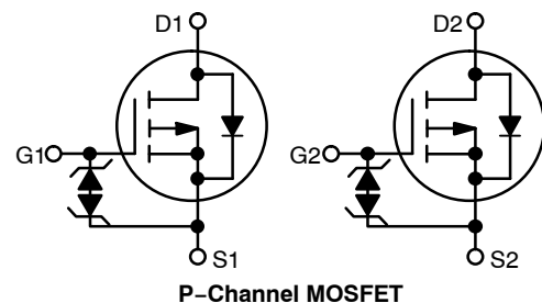
P-Channel MOSFET
