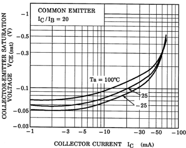
Fig. 10.11 RN2908 V_{CE(sat)}-I_C
