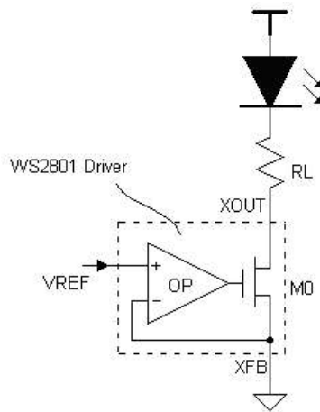
Fig4, 恒定电压驱动模式电路示意图
