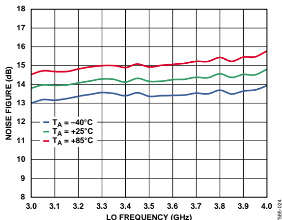
图24. 噪声系数与LO频率的关系
