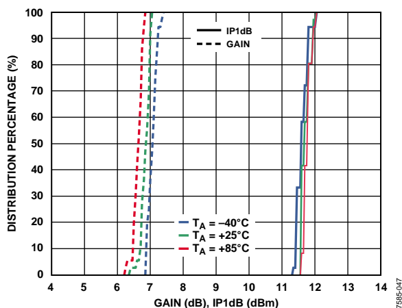
图47. 增益和IP1dB分布
