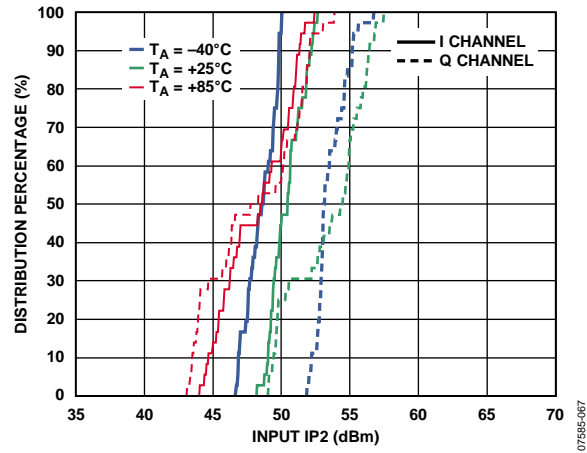
图67. I通道和Q通道的IIP2分配
