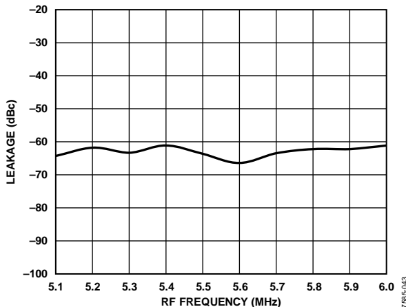
图43. RF至LO泄漏与RF频率的关系
