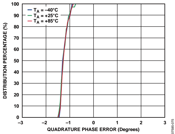
图75. IQ正交相位误差分配
