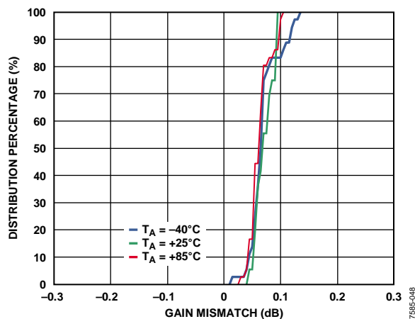
图48. IQ增益失配分布
