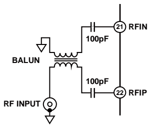
图79. RF输入
