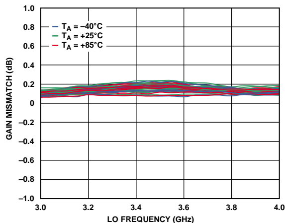
图22. IQ增益失配与LO频率的关系
