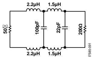
图92. 四阶低通LTE滤波器原理图
