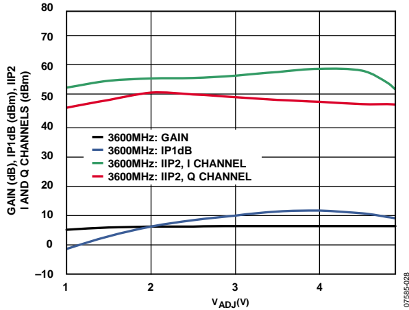
图28. 转换增益、IP1dB和IIP2与 V_{ADJ} 的关系, f_{LO} = 3600\text{ MHz}
