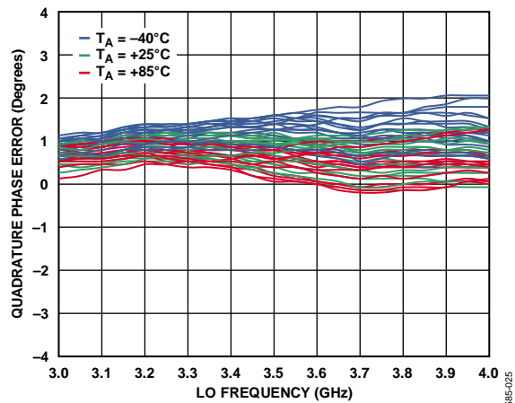
图25. IQ正交相位误差与LO频率的关系
