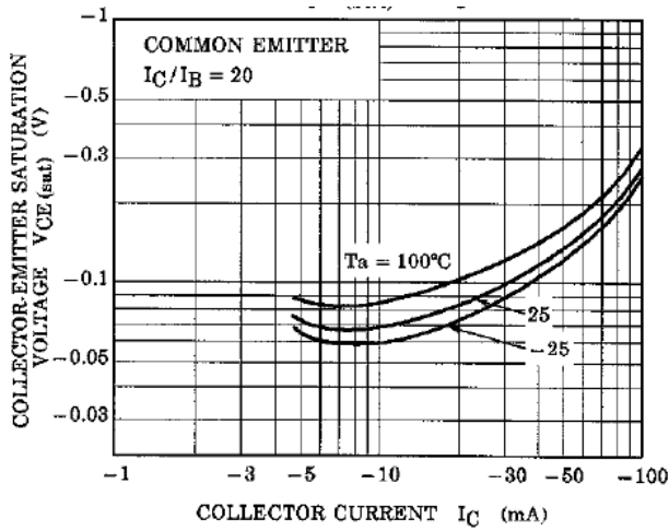
Fig. 10.19 RN2901 V_{CE(sat)}-I_C
