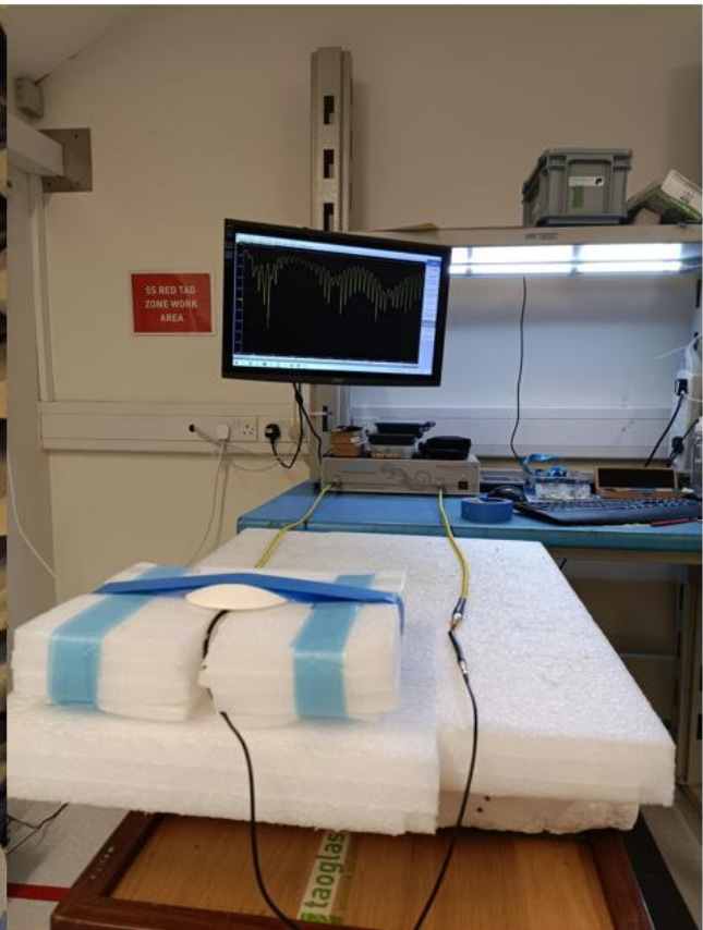
VNA Set up
