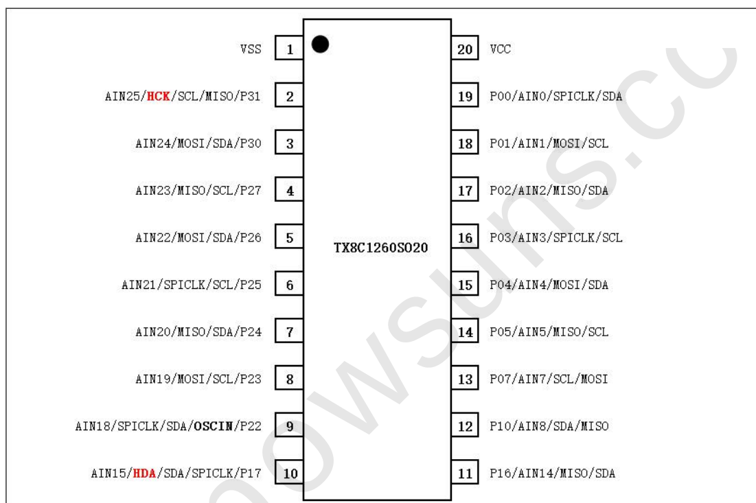
图 5 - TX8C1260SO20 (SOP20) 封装图
