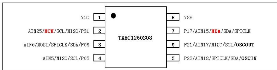
图 4 - TX8C1260SO8 (SOP8) 封装图
