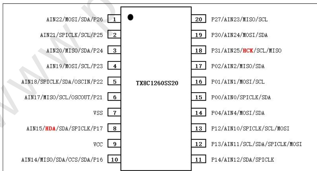
图 3 - TX8C1260SS20 (SSOP20) 封装图
