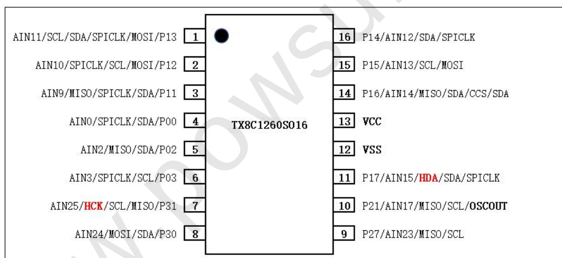
图 7 - TX8C1260SO16 (SOP16) 封装图
