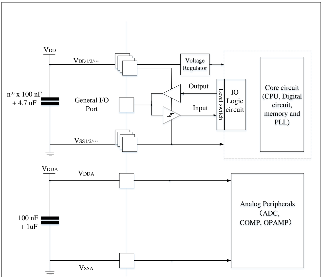
图 4-3 供电方案
