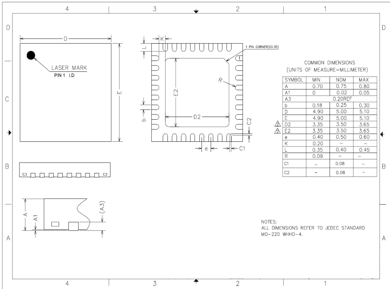
图 5-3 QFN32(5mx5m)封装尺寸
