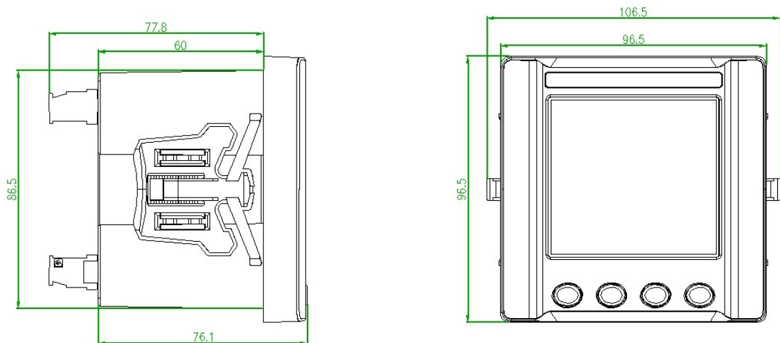
图 1 APM510 尺寸图
