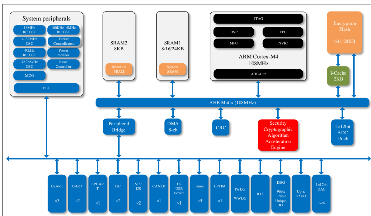
图 1-1 N32G432 系列框图
