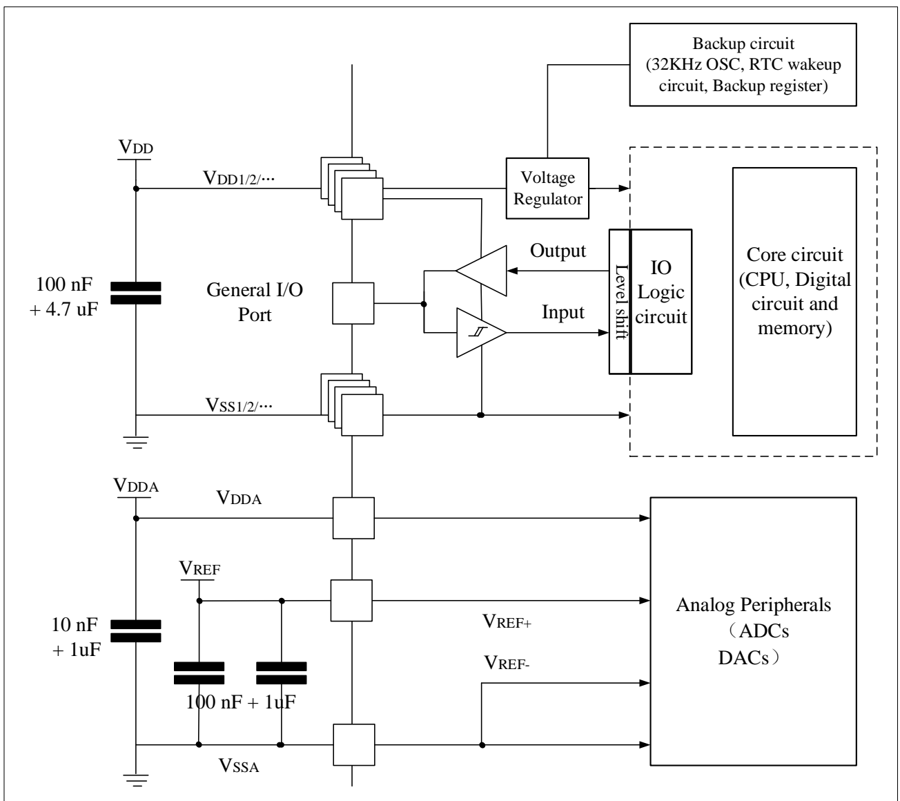
图 4-3 供电方案
