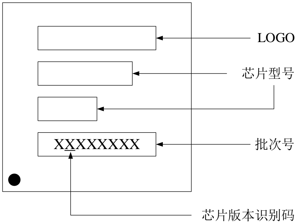
图 5-4 丝印说明
