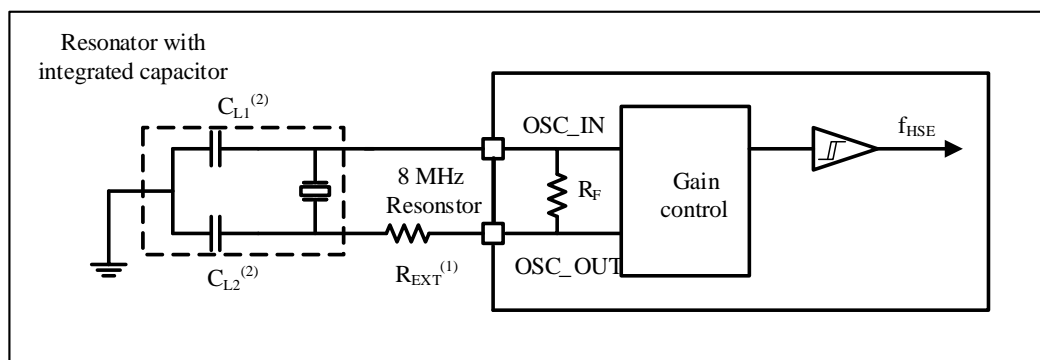
图 4-7 使用 8MHz 晶体的典型应用
