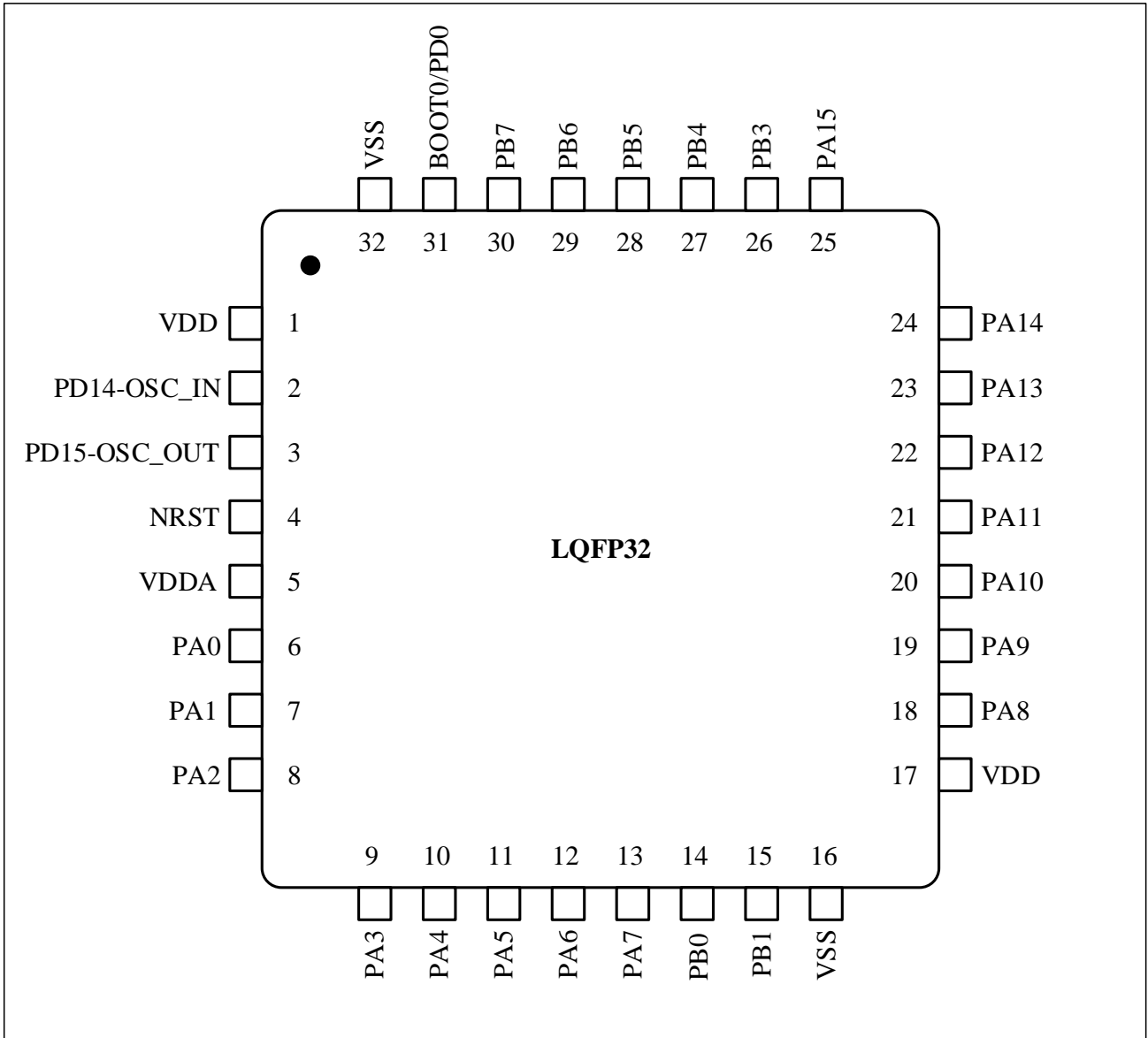
图 3-1 N32G432 系列 LQFP32 引脚分布
