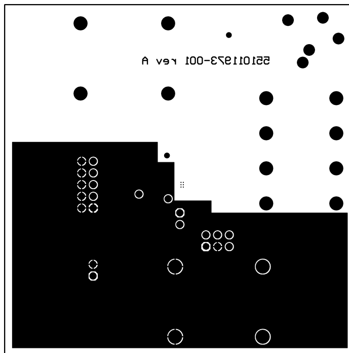
Figure 26. Bottom Layer
