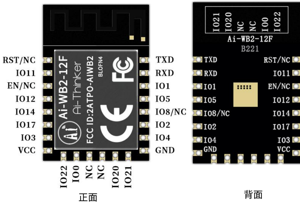
图 6 管脚示意图
