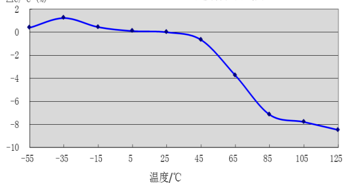
TCC0603X7R104K500CT-温度特性曲线图
