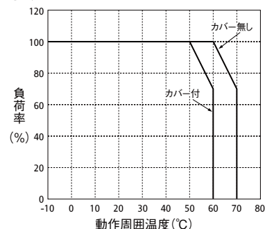
強制空冷時の 出力デイレート
