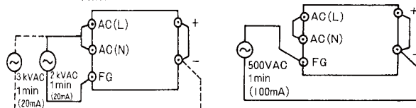
入力-FG間(実線) 入力-出力間(破線)
