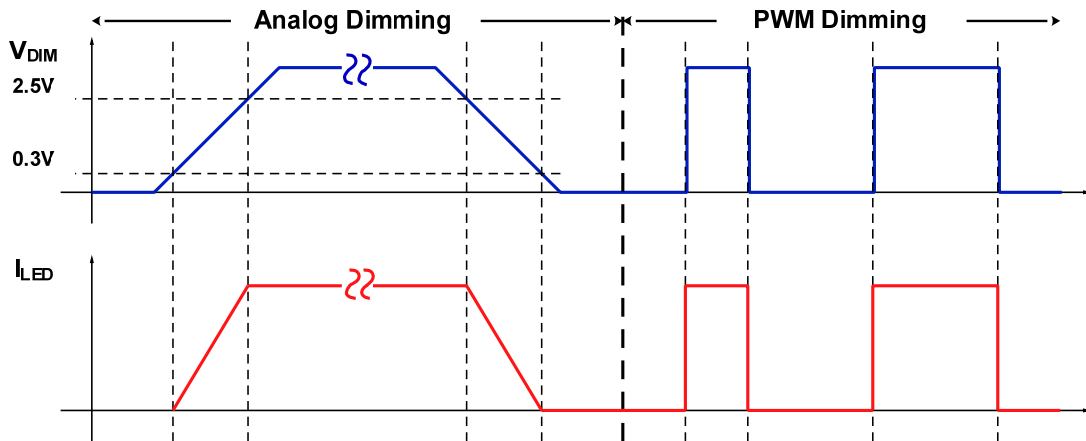
图 14. 调光波形示意图
