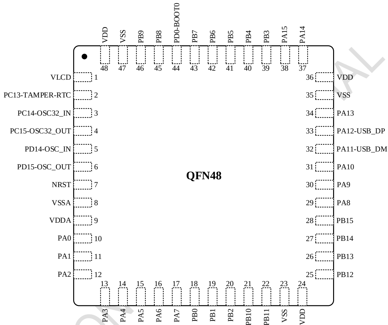
图 3-2 N32L406系列QFN48引脚分布
