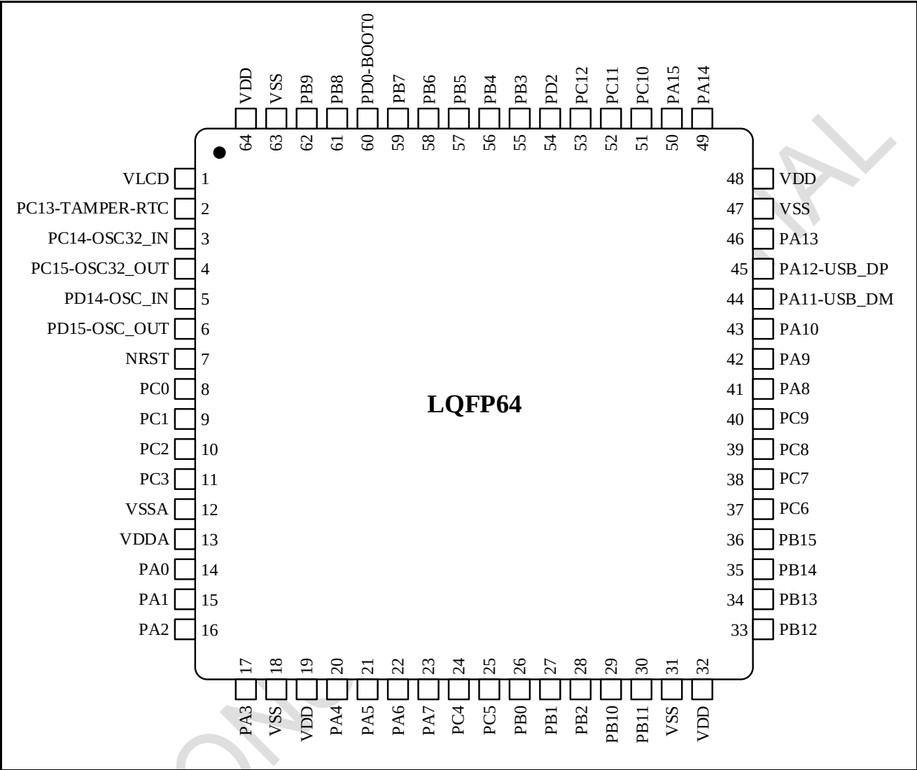
图 3-7 N32L406系列LQFP64引脚分布
