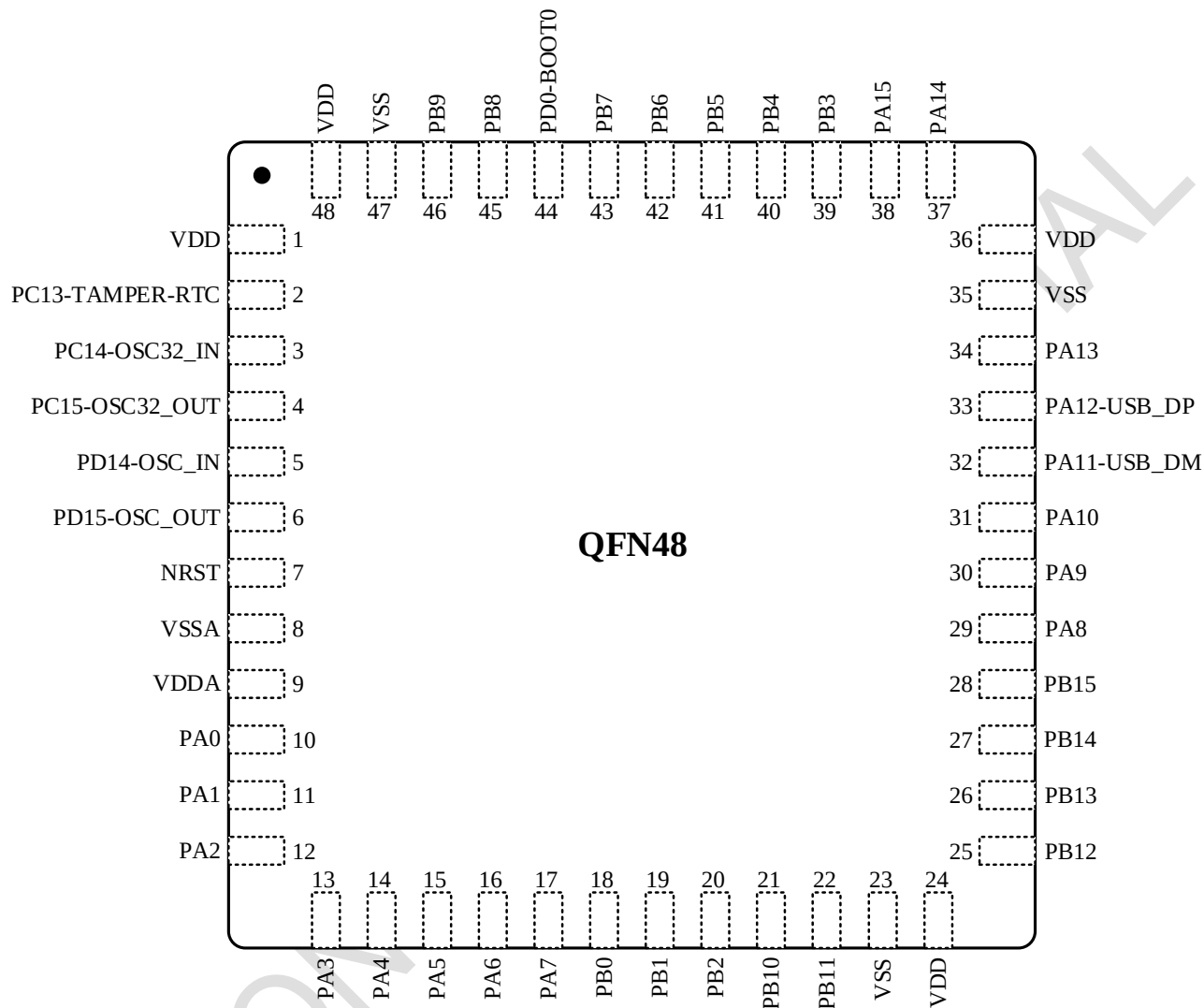
图 3-3 N32L401系列QFN48引脚分布
