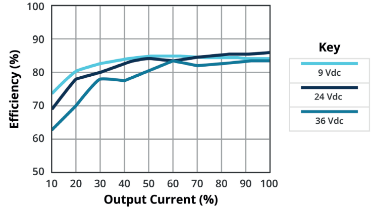
EFFICIENCY VS OUTPUT LOAD PDQ15-Q24-D5-D
