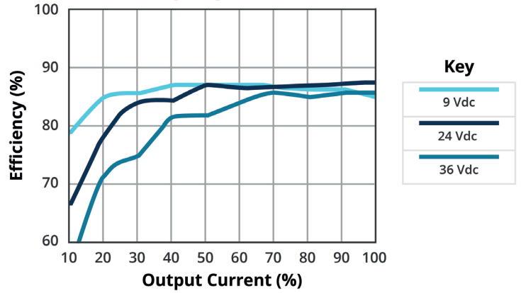
EFFICIENCY VS OUTPUT LOAD PDQ15-Q24-D5-D
