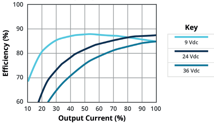
EFFICIENCY VS OUTPUT LOAD PDQ15-Q24-S15-D
