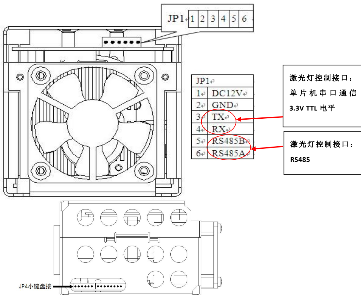
JDD-800-HD 产品的接口管脚分配图
