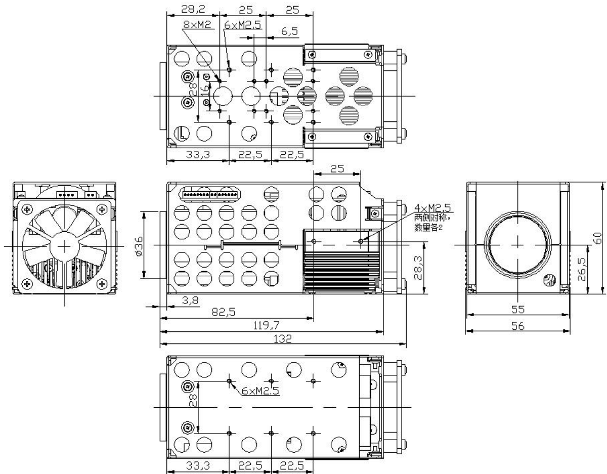
JDD-1000-HDX 结构尺寸图
