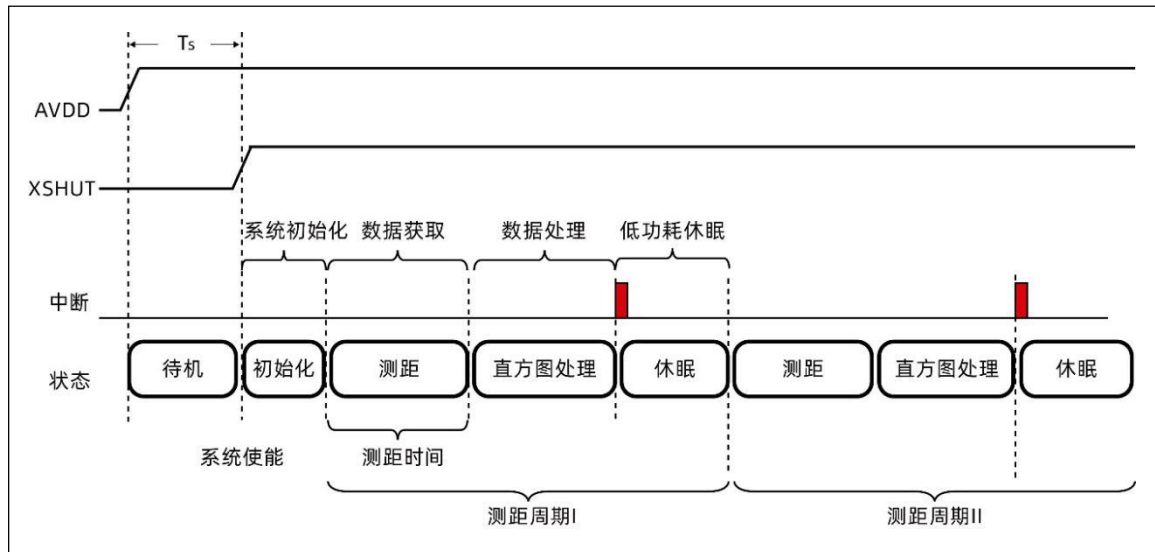
测距时序图
