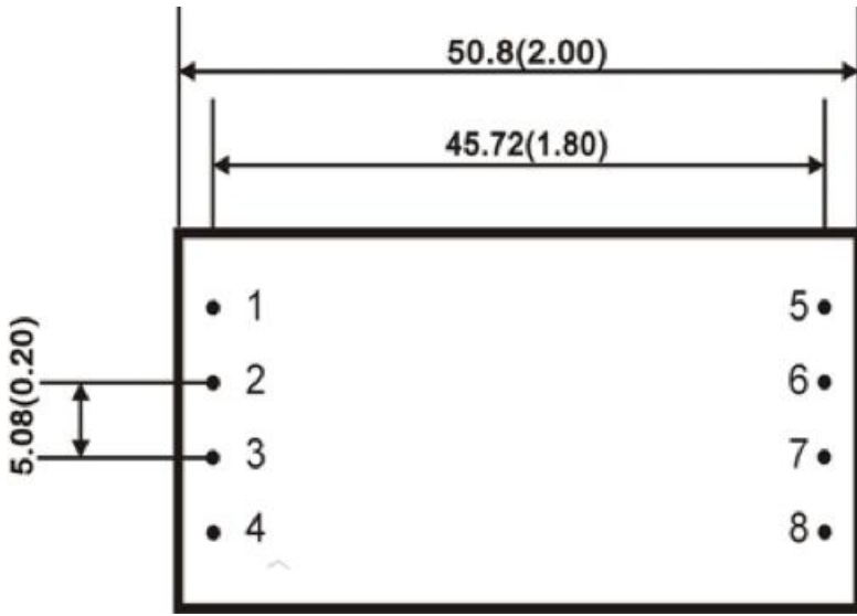
底视图
