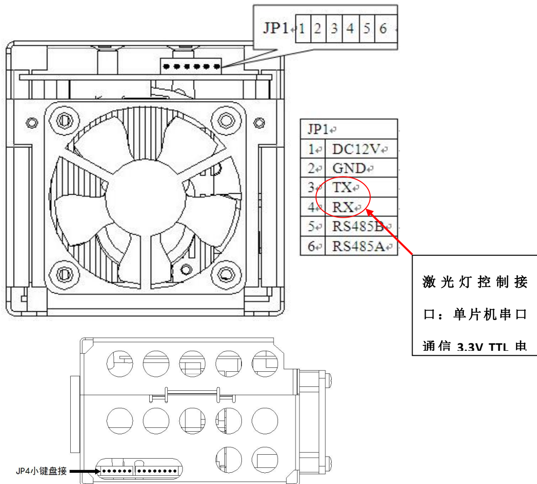
JDD-500-HD 产品的接口管脚分配图
