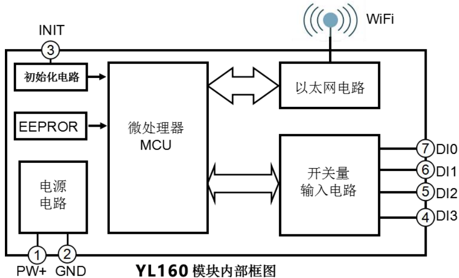
图 2 YL160 模块内部框图
