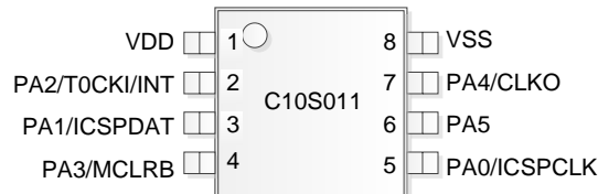
图 1.5 SOP-8 脚位图
