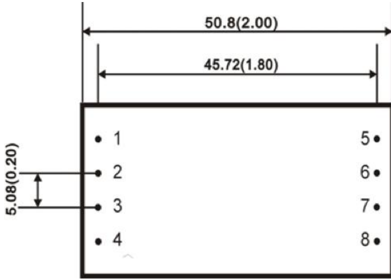
底视图
