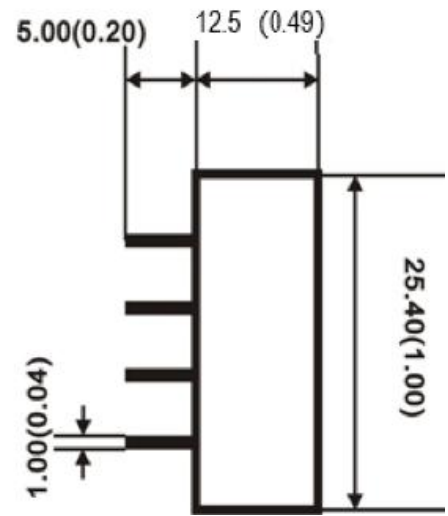
侧视图
