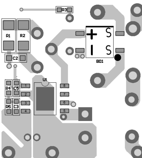
Bottom Layer
