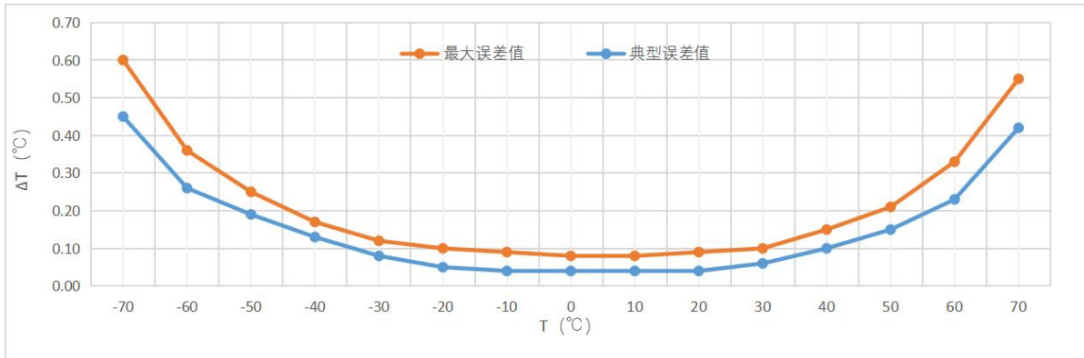
图 7-4 M117P 精度误差曲线
