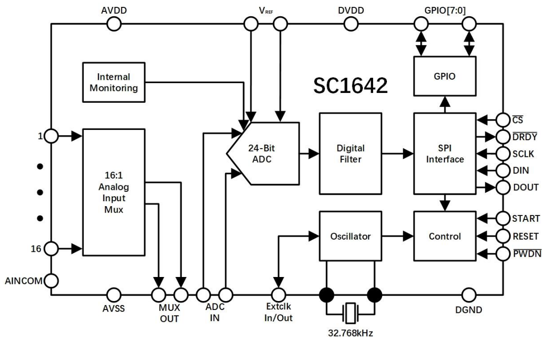
图 1 芯片模块示意图
