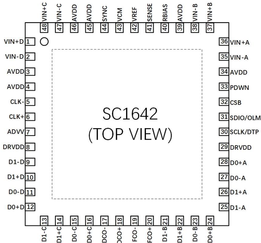
图 2 管脚（焊盘）配置
