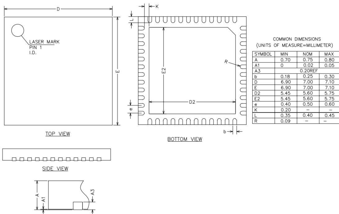
图 36 48 脚 QFN 封装尺寸图
